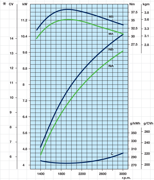
KDW702/B1 @ 3000 RPM
