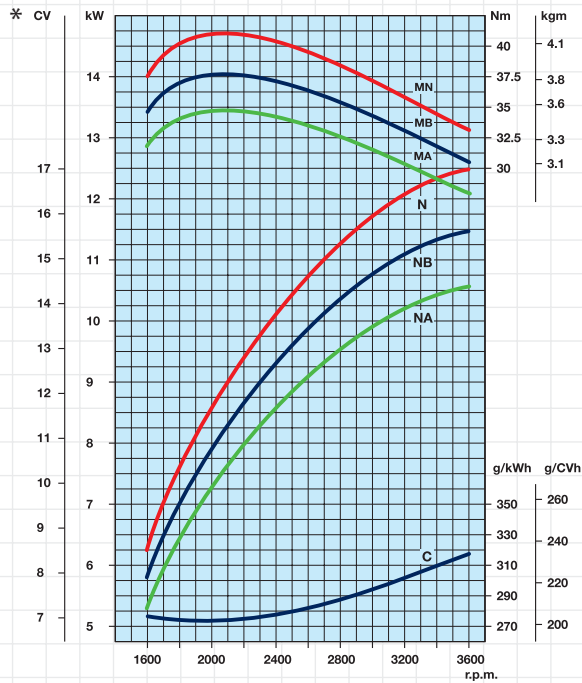
KDW702 @ 3200 RPM
